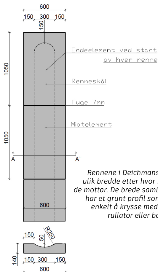
Bruk av Aco Drain i områder der avrenningen har med seg mye sedimenter øker faren for at renna går tett eller gror igjen.
